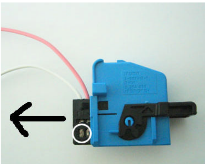
Bild 3: Steckergehäuse entfernen
