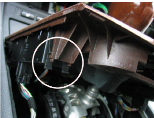
Bild 7: Fensterheberschalter
